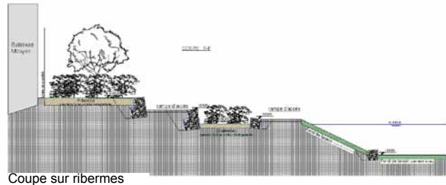
Coupe sur riberms
